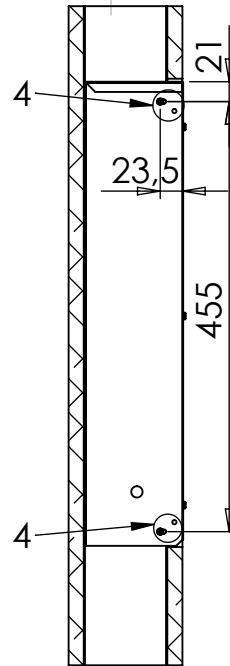
SEZIONE F-F SCALA 1 : 8
