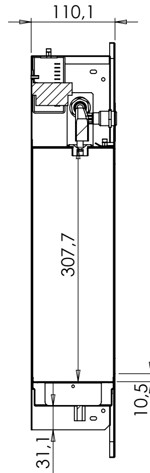
SEZIONE E-E SCALA 1 : 5
