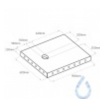
Żelbetonowa płyta fundamentowa, montażowa 900*600*150 mm, masa 190 kg 196.960.366
